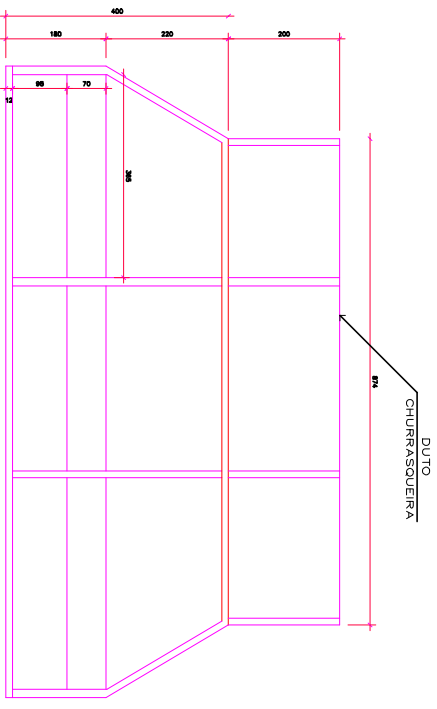
CORTE A - A' Esc: 1/90
