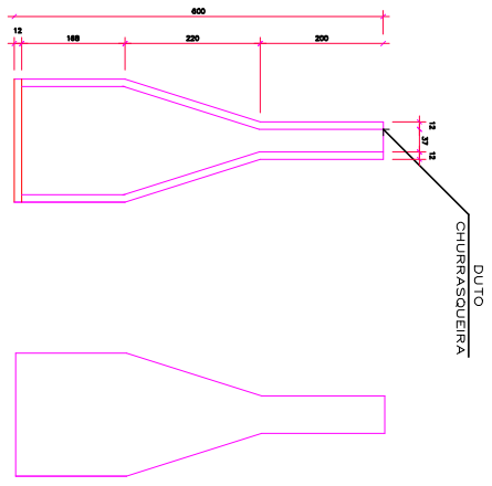
CORTE B - B' Esc: 1/90
