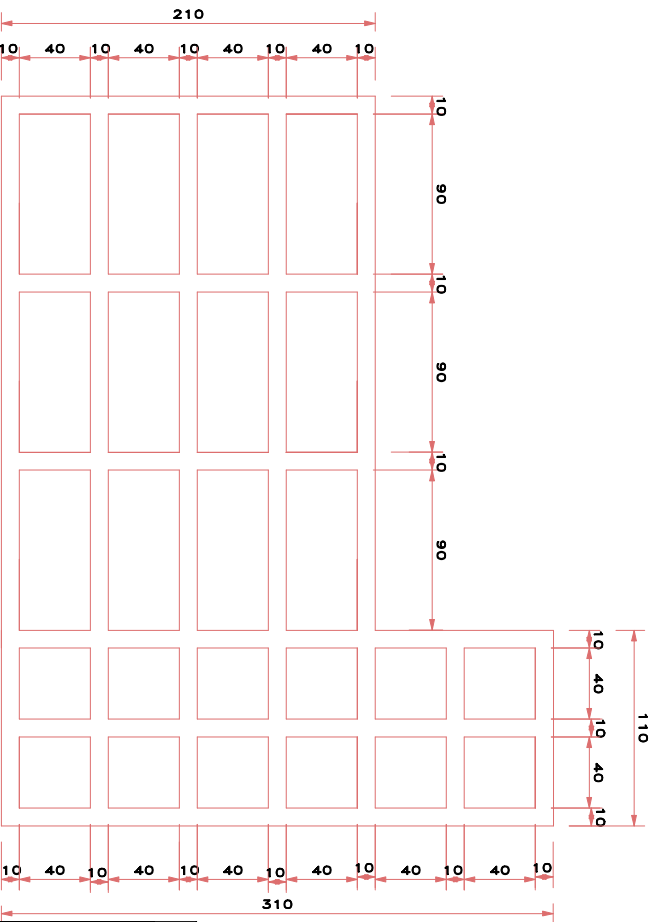
CORTE A-A', ESC: 1/50
