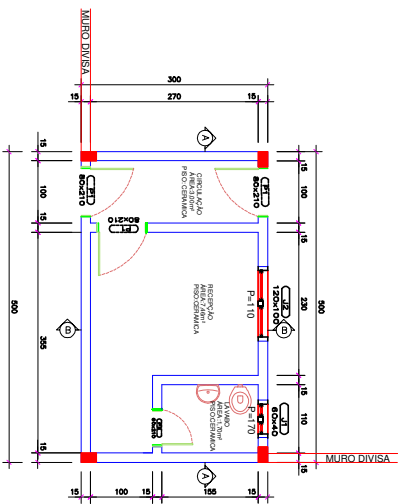
PLANTA BAIXA Escala 1/50 A:15,00 m 2
