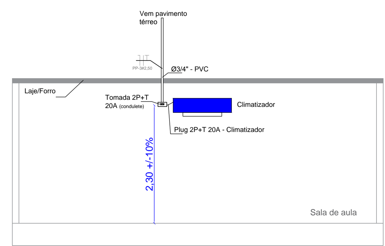
DETALHE INSTALAÇÃO DO CLIMATIZADOR SEM ESCALA
