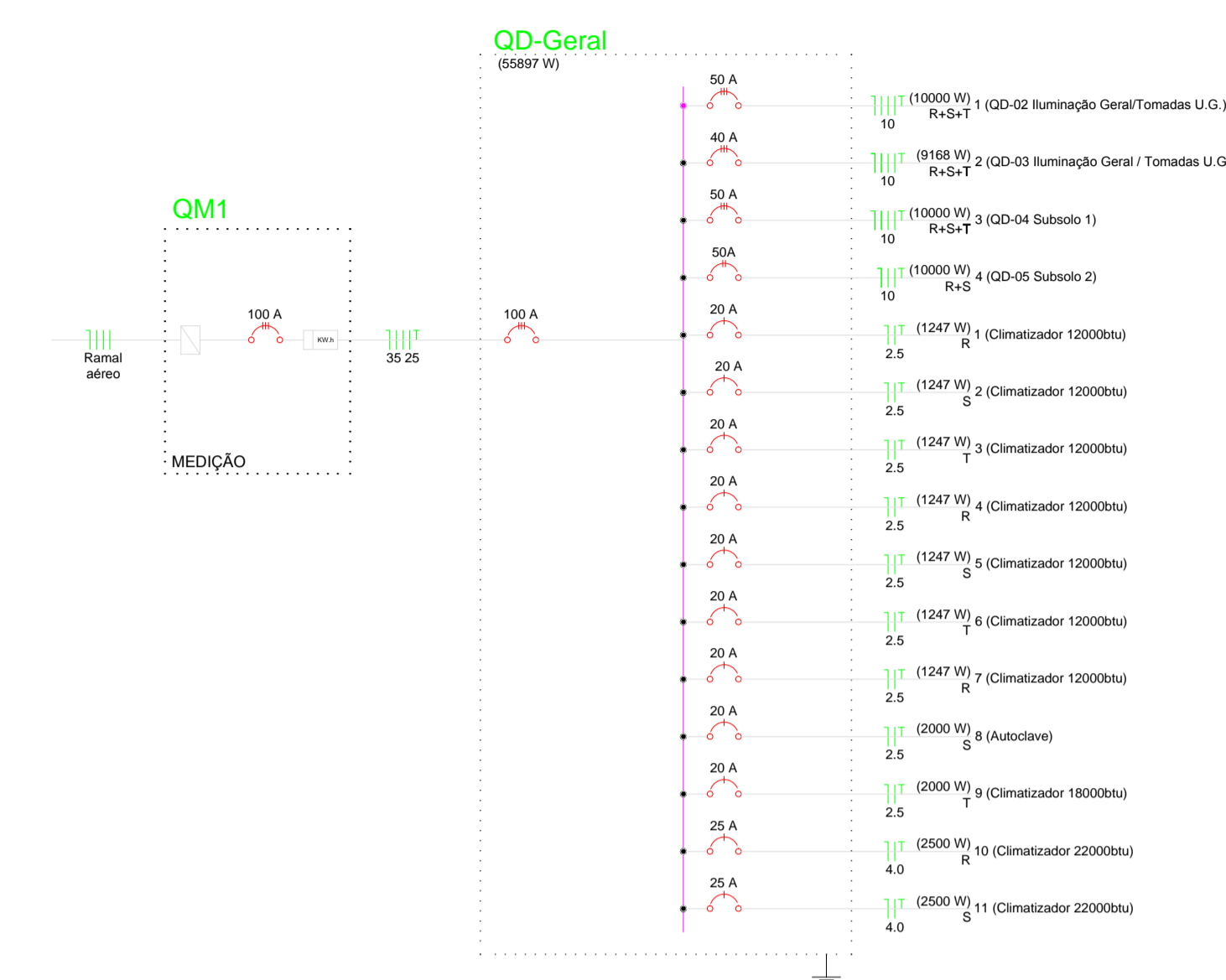
DIAGRAMA UNIFILAR SEM ESCALA
